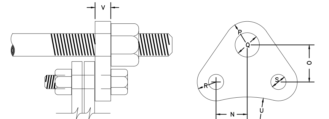
FLANGE LUG DETAIL
