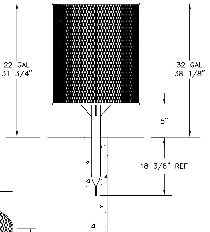
RECEPTACLE DIMENSIONS
